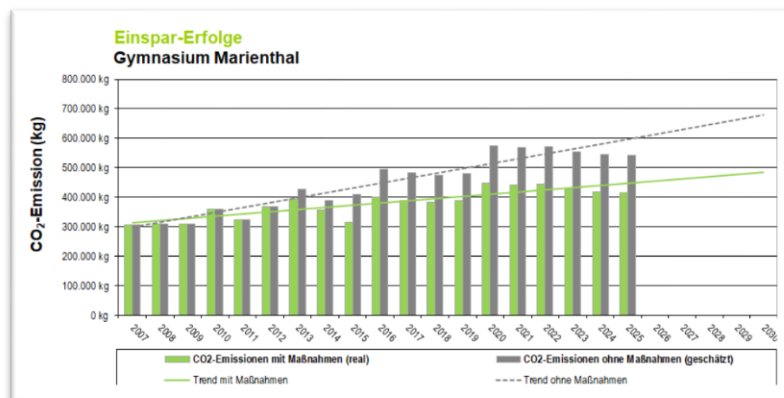
Diagramm 3: Erfolge dank Maßnahmen
